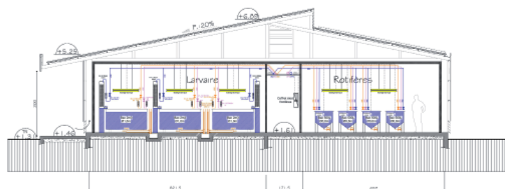
BATIMENT ECLOSERIE POISSONS COUPE DE PRINCIPE HYDRAULIQUE
