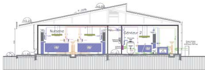
BATIMENT ECLOSERIE POISSONS COUPE DE PRINCIPE HYDRAULIQUE
